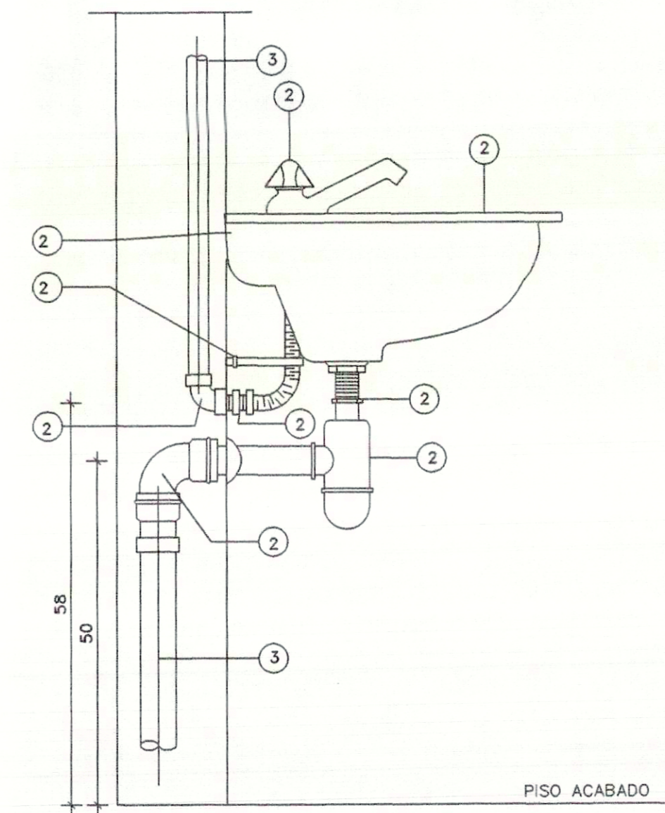
DETALHE DE INSTALAÇÃO DO LAVATORIO INDIVIDUAL ESCALA 1:20
