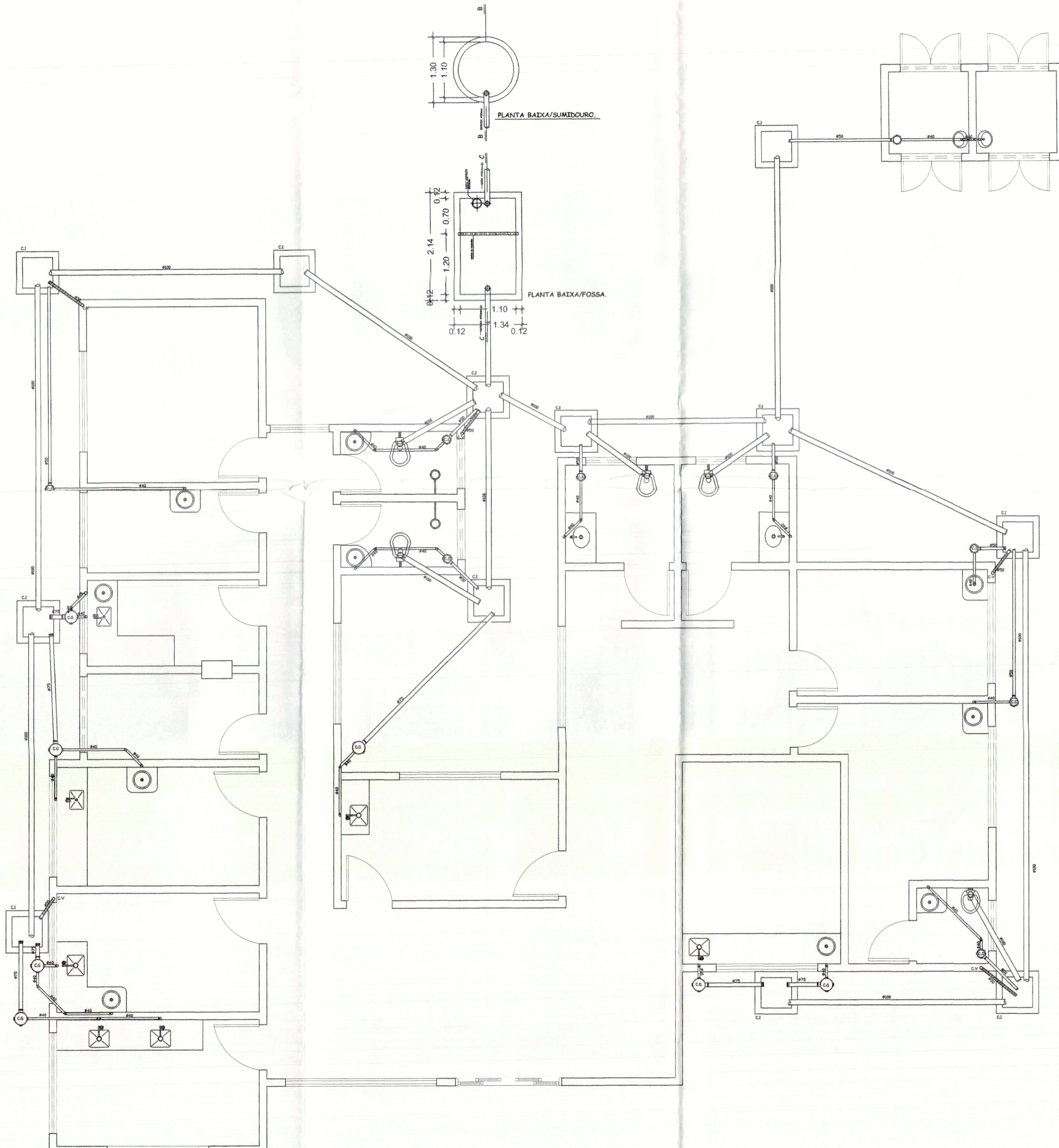
SANITÁRIO ESCALA 1:50
